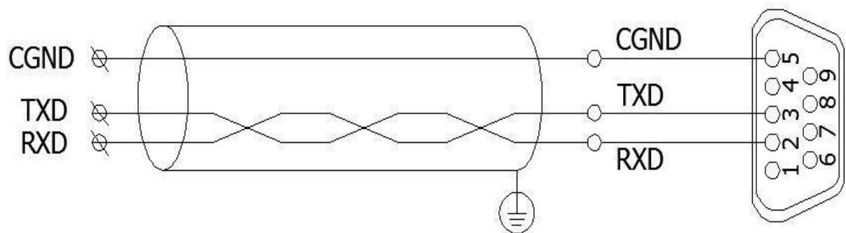
仪表外置RS232C通讯接线端子
