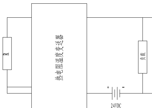
图 3 WTYYS-1* 1 * 2 * 3 -□□接线图
