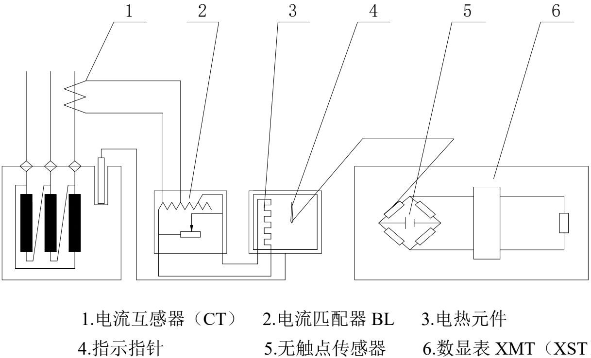
图 2 工作原理图
