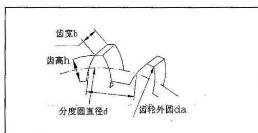
图四 测速齿轮结构图
