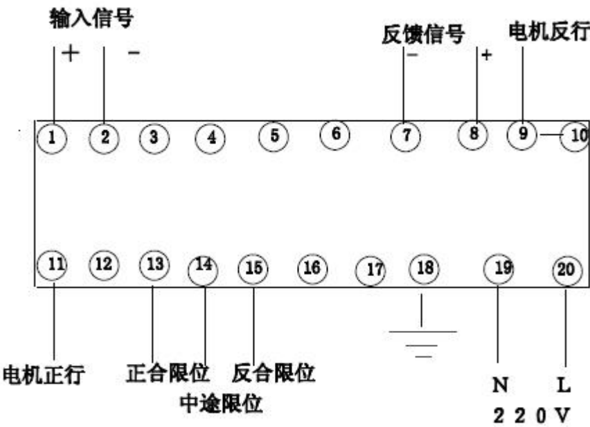
ZPE-2030QII\III 伺服放大器接线端子图
