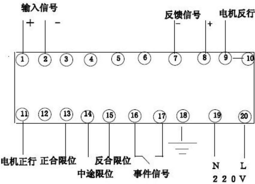
ZPE-2031QIII 伺服放大器接线端子图
