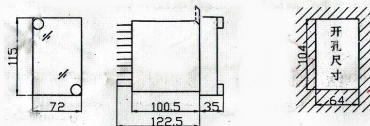
外形尺寸图
