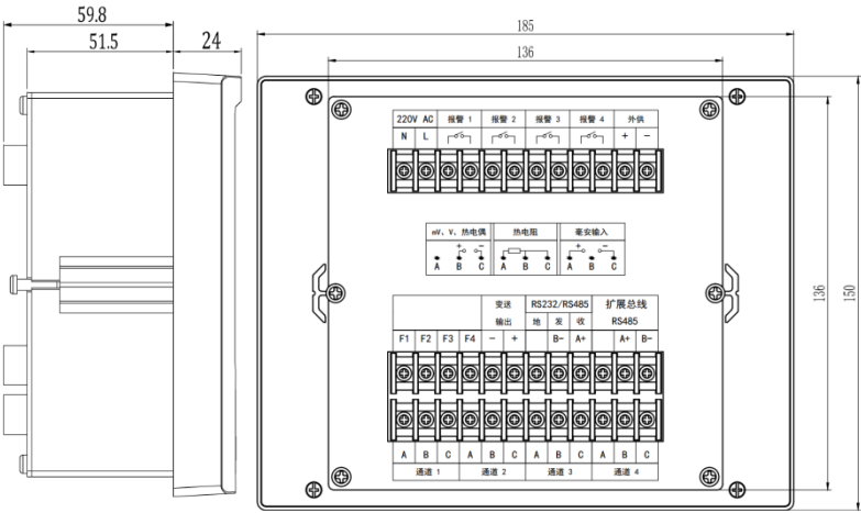
开孔尺寸
