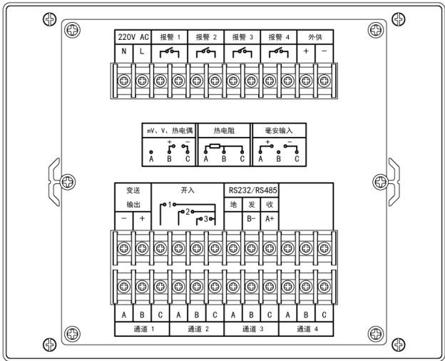
图 2.3.1.1 后端子图
