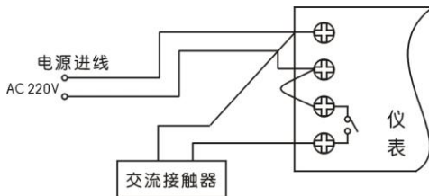
错误接法
