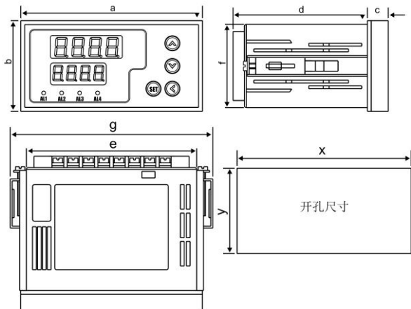
96×48 尺寸仪表
